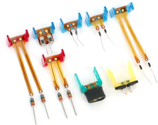
Tip-Clip assemblies
